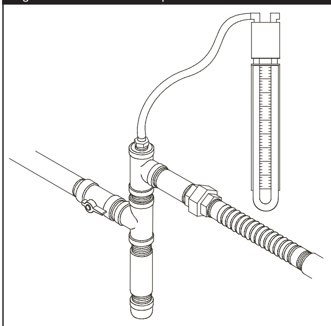
Figure 33 — Manomètre Temporaire Installé
